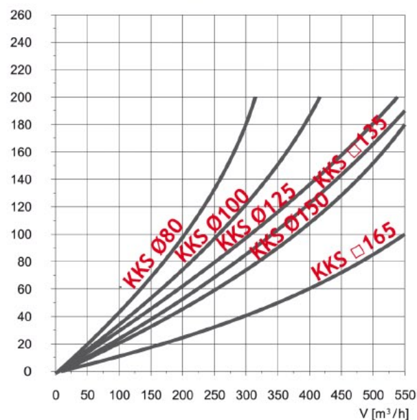
Graf tlakové ztráty
