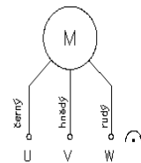
SMYSL TOČENÍ PŘI POHLEDU NA VÝSTUPNÍ HRDEL PŘEVODOVKY (REVERZACE JE MOŽNÁ PŘEPOJENÍM DVOU LIBOVOLNÝCH VÝVODŮ)
