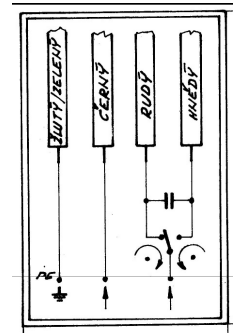
Kondenzátor 4µF/260V
