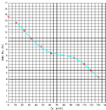
Charakterystyka wydajności wentylatora Charakteristika ventilátoru Charakteristika ventilátora
