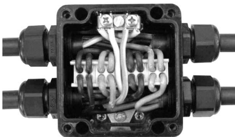
Příklad zapojení 4 kabelů CYKY 5C × 2,5 mm 2
