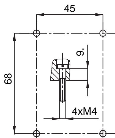
Upevňovací otvory
