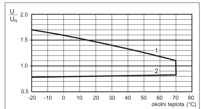
R 66 - pracovní rozsah AC cívky
