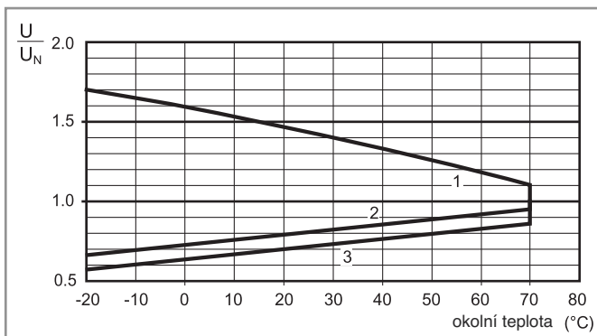
R 66 - pracovní rozsah DC cívky
