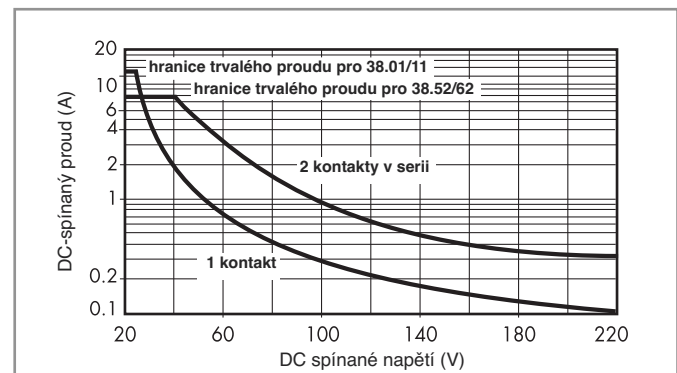
H 38 - spínací schopnost při DC1, 1P / 16 A a 2P / 8 A
