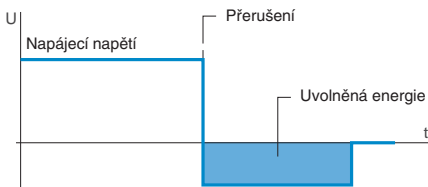
Napětí cívky s modulem ochranné diody ( \text{---} pouze)
