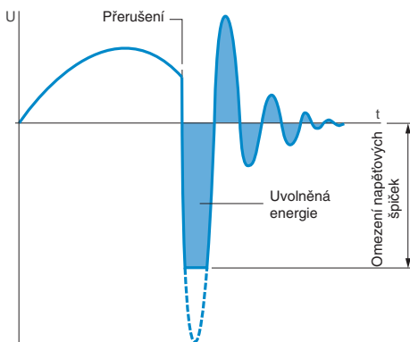
Napětí cívky s modulem varistoru ( \sim a \text{---} )
