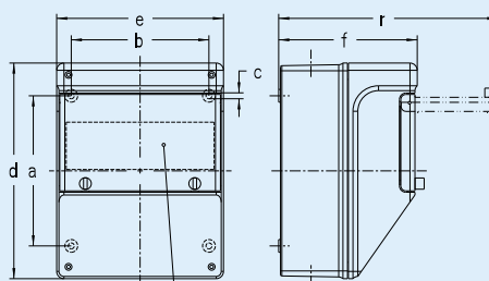
Typ 692 – s otvorem
