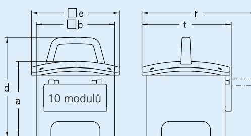
Typ 649 – s otvorem
