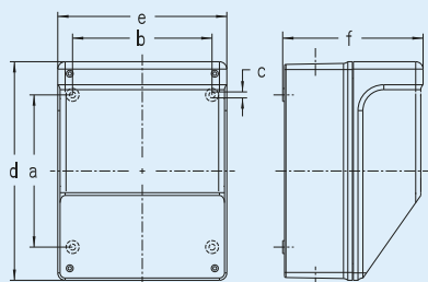
Typ 691 – bez otvoru
