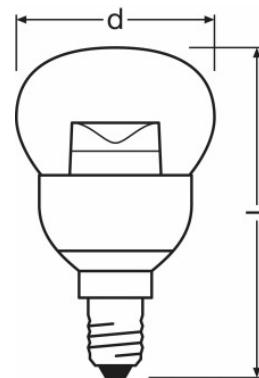
PARATHOM CL P 25 4 W/827 CD E14
