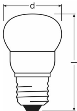
PARATHOM CL P 25 4 W/827 FR E27
