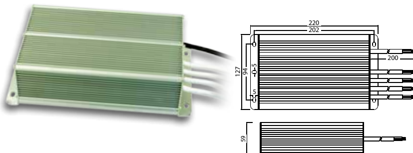
7 Napájecí zdroj 200W IP67
