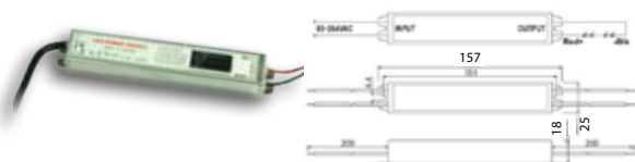
3 Napájecí zdroj 40W IP67
