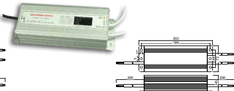
7 Napájecí zdroj 200W IP67
