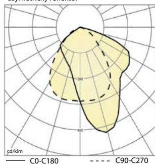
XANTI-400H, 1x400W, IP65 - asymetrický reflektor
