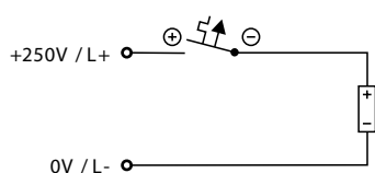
Příklad zapojení při 250 V, 1pólové
