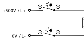
Příklad zapojení při 500 V, 2pólové
