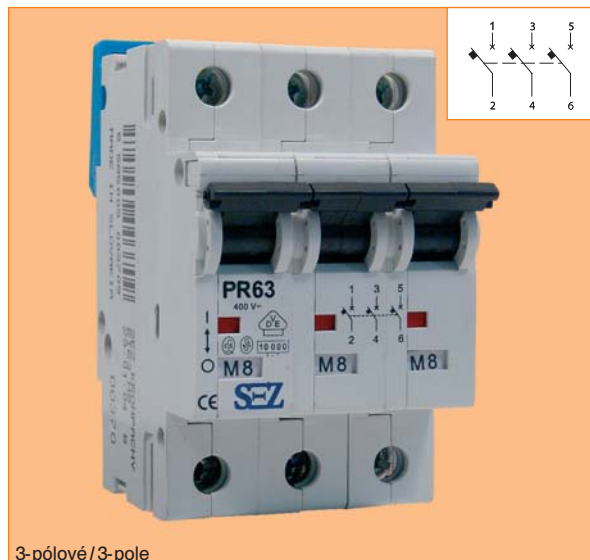
3-pólové / 3-pole
