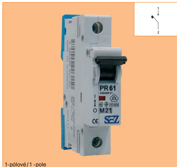
1-pólové / 1 -pole
