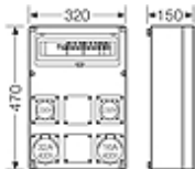
rozměrový výkres
