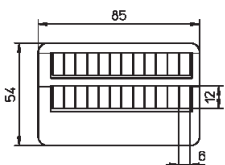
NO-6x12 120 Mini - štítky
