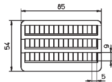
NO-5x9 225 Mini - štítky
